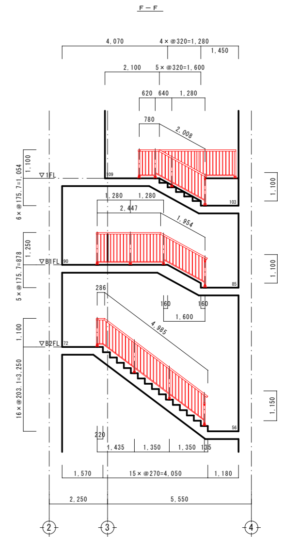
改修後立面図
