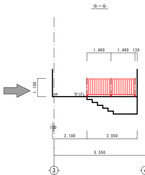
改修後立面図
