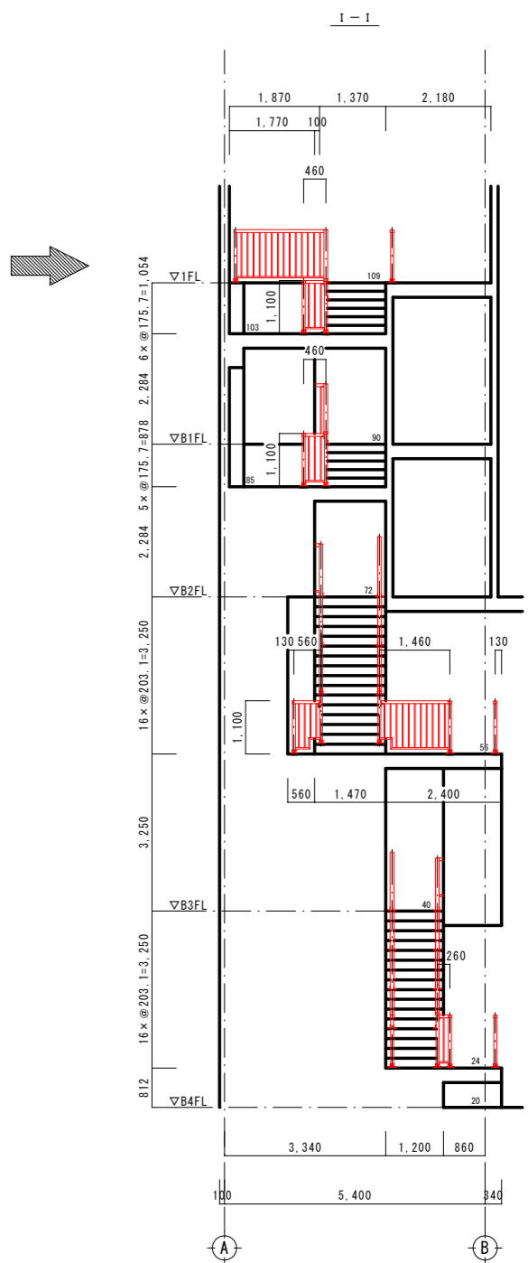
改修後立面図
