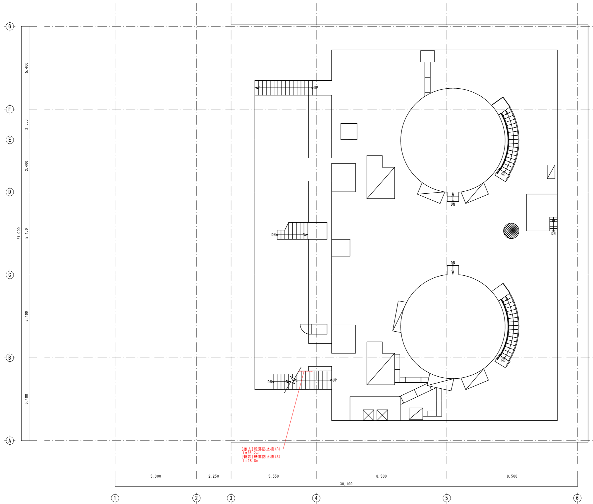
B 5階平面図 S=1/100
