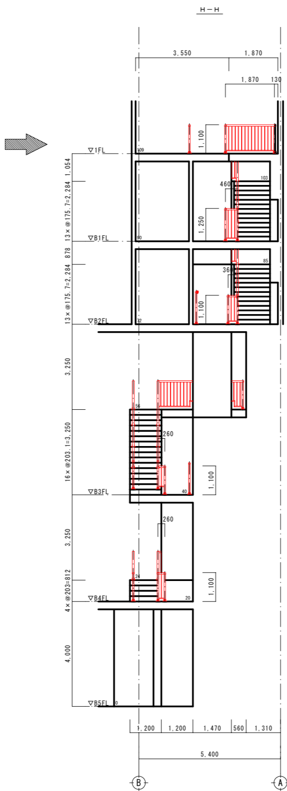
転落防止柵詳細図(5) S=1/100
