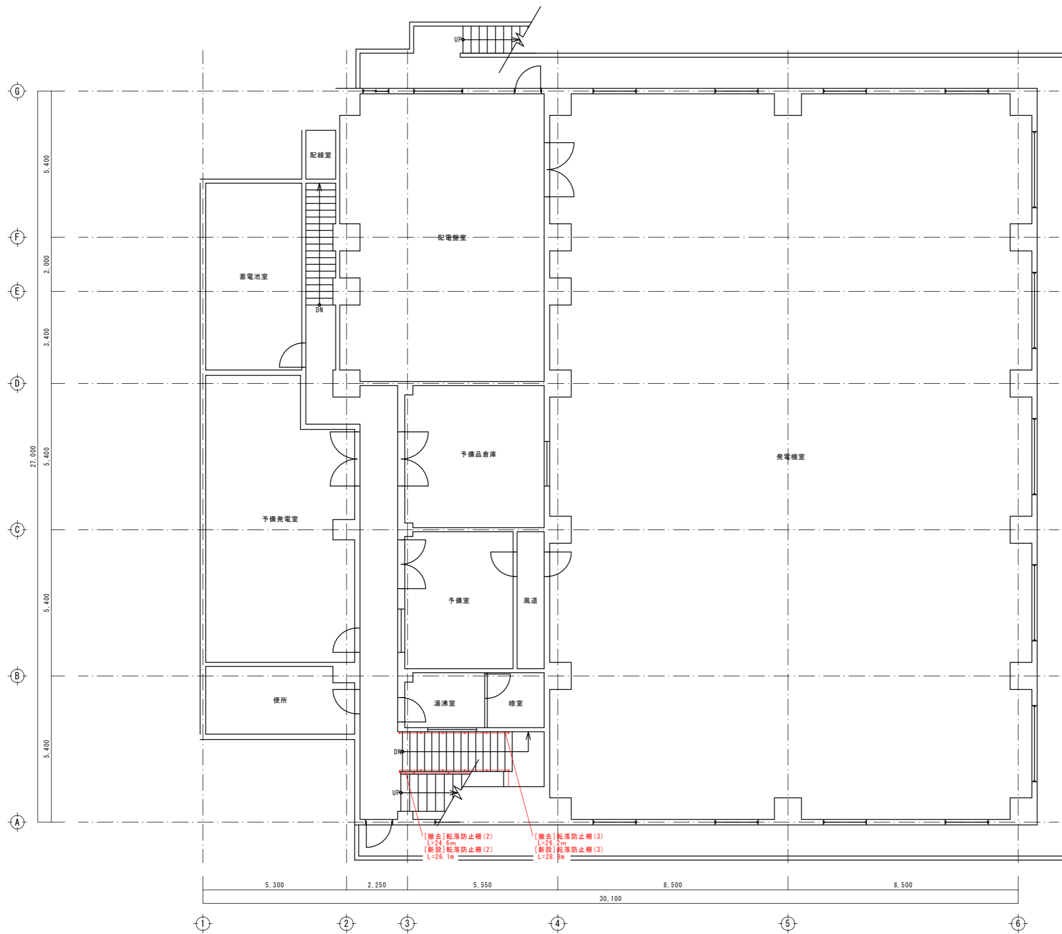
B 2 階平面図 S=1/100
