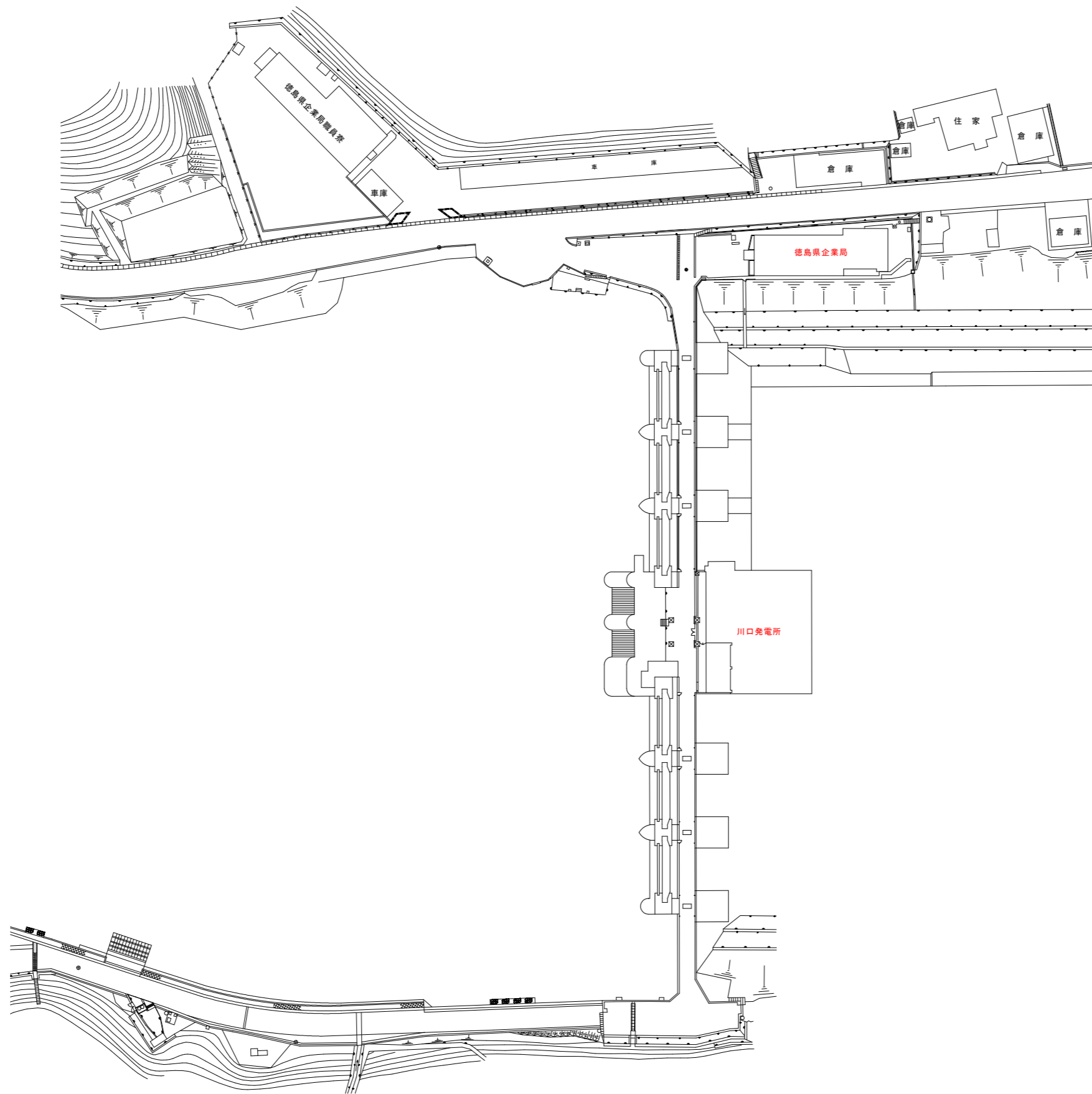
全体配置図 S=1/750
