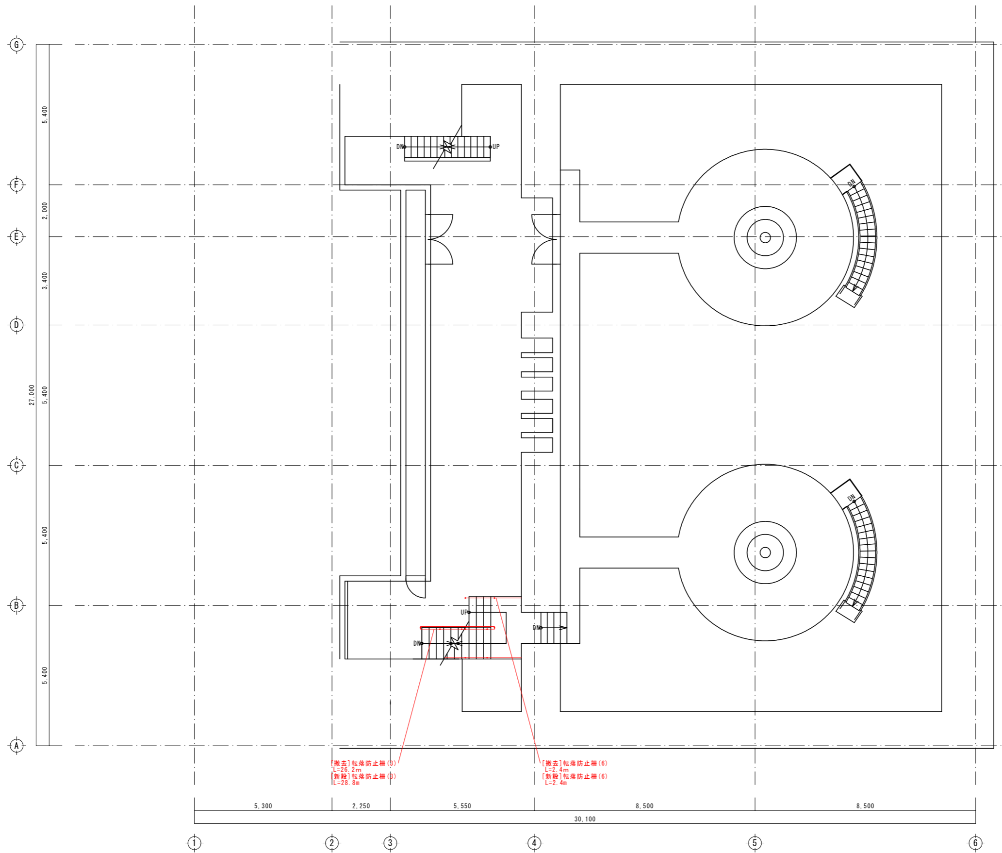
B 4 階平面図 S=1/100
